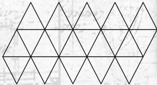
desfasurata icosaedrului
